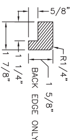
DETAIL -C SCALE: 3"=1'-0"
